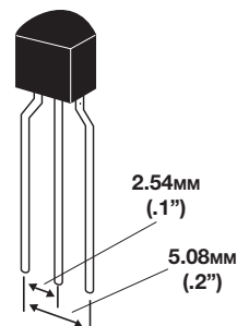
TO92T-.2
