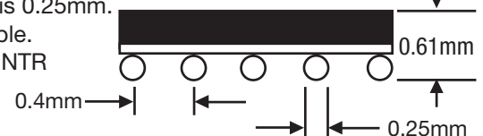
WLP676T.4C-DC260D
