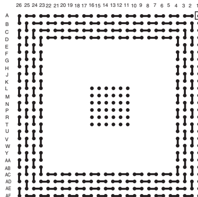
BGA388T1.27-DC72
