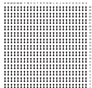
WLP676T.5C-DC260D
