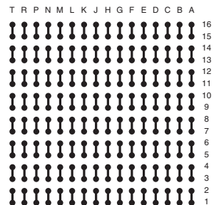
WLP256T.5C-DC168D
