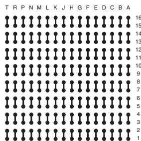
WLP256T.4C-DC168D
