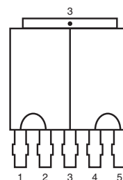
DC1245 D2PAK5
