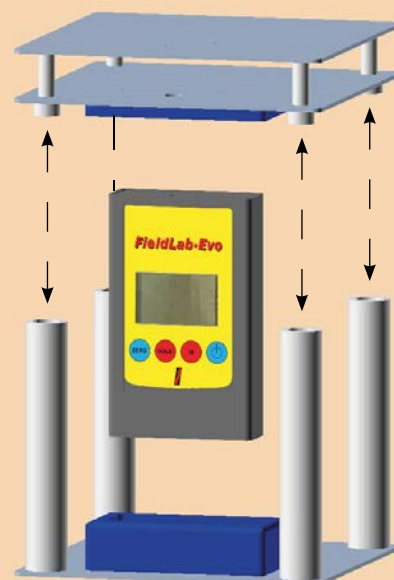
FieldLab Evo con opzione 9265.705 (Charge Plate Monitor)
